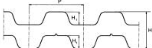
T5 DL - T10 DL - T20 DL
