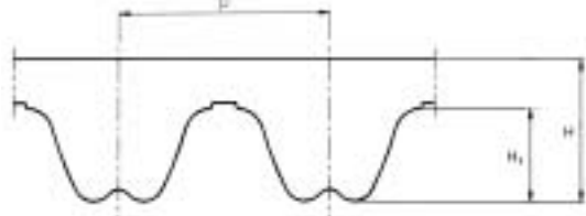
RPP5 - RPP8 - RPP14
