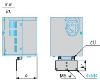
(1) 2 x M5 screws
