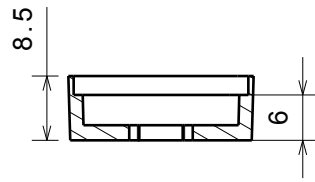
Section view C-C Scale: 1:1
