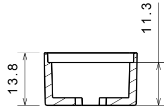
Section view B-B Scale: 1:1
