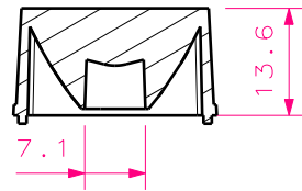
Section view B-B Scale: 1:1
