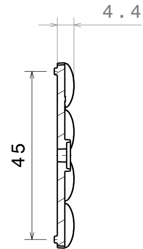
Section view A-A Scale: 1:1
