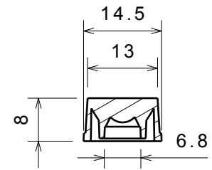
Section view B-B Scale: 1:1
