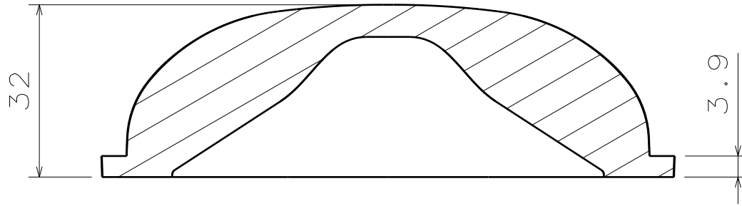
Section view A-A Scale: 1:1
