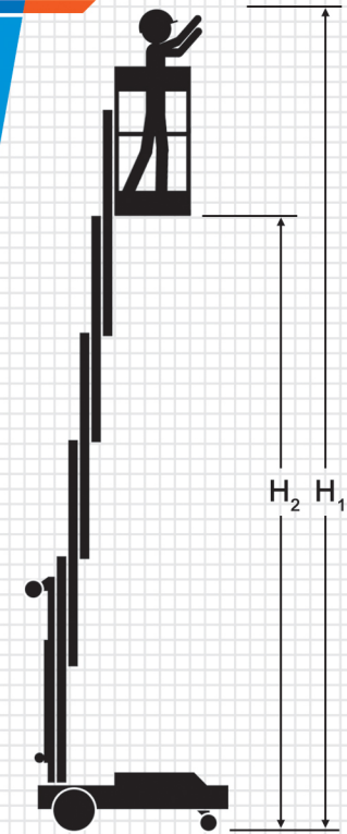
نمای جانبی دستگاه در حالت باز شده Side view in unfolded status
